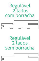
BATENTE Regulável 2 lados
